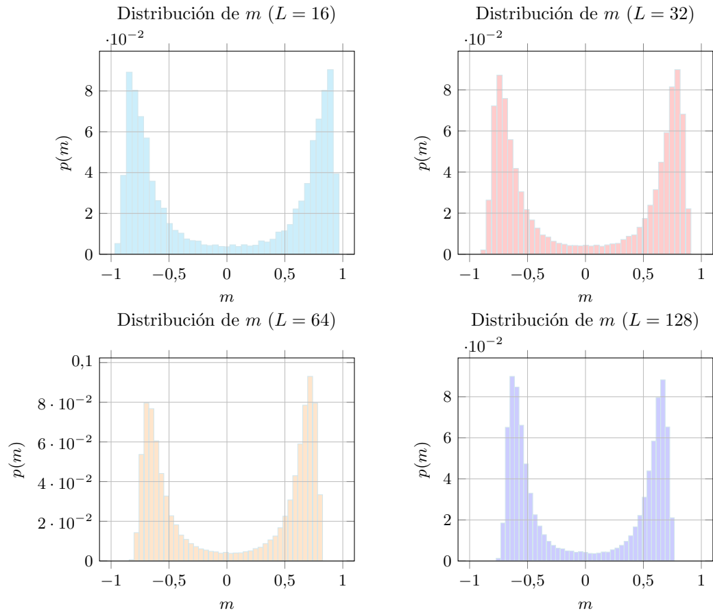
Figura 2: Densidad de probabilidad de la magnetización m en \beta_{crit}
