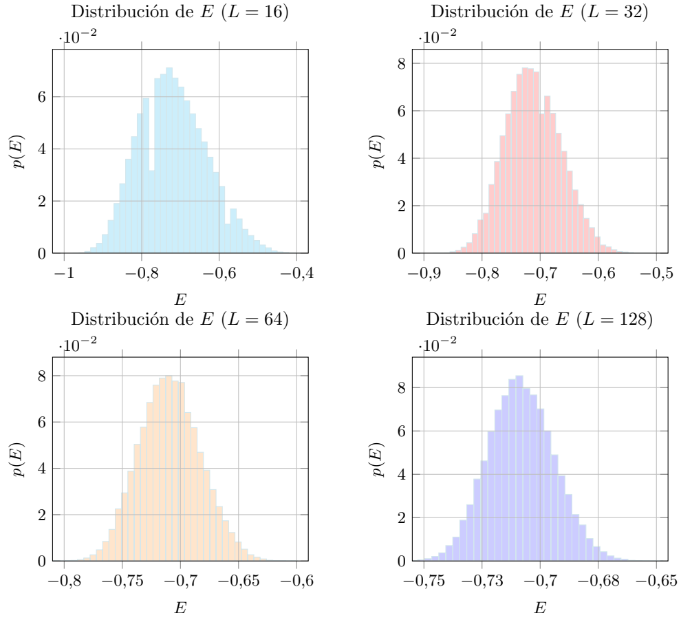
Figura 1: Densidad de probabilidad de la energía E en \beta_{crit}
